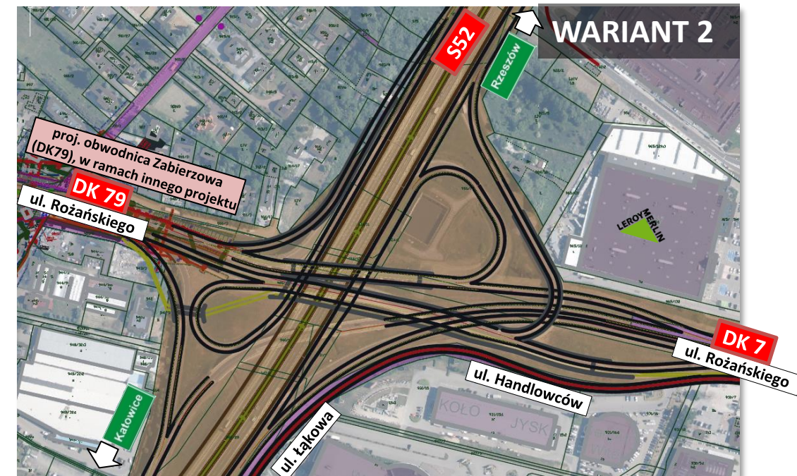
Węzeł Modlniczka propozycje wariantów węzłów
